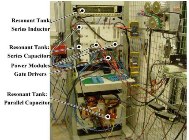
Fig. 16. Test setup.
