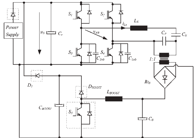
Fig. 17. Test setup circuit diagram.
